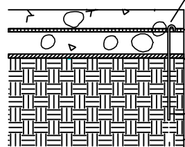
ДЕТАЙЛ А
